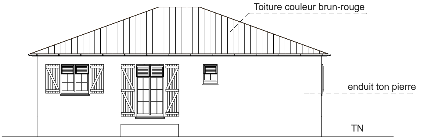
FACADE Nord
